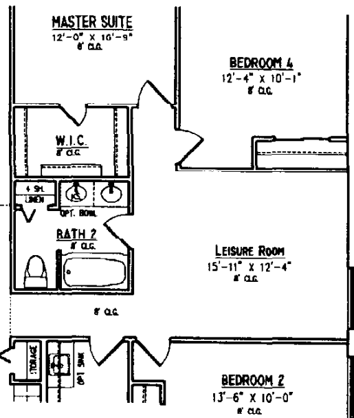
OPTIONAL LEISURE ROOM IN LIEU OF BEDROOM 3 RMS 02200
